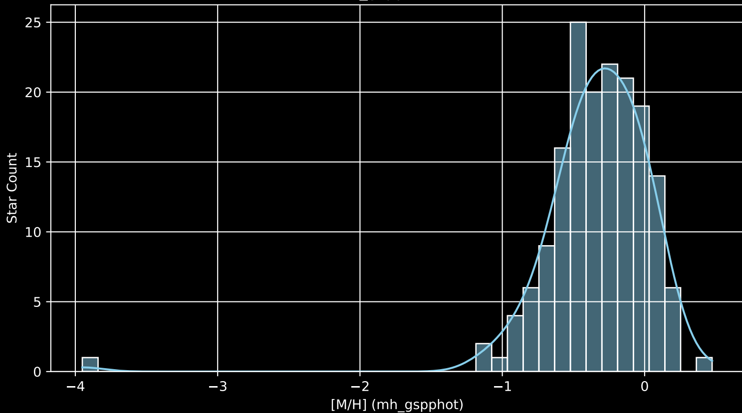
GALAH DR4 Field: [7205] [M/H] (mh_gspphot) (n= 167)
