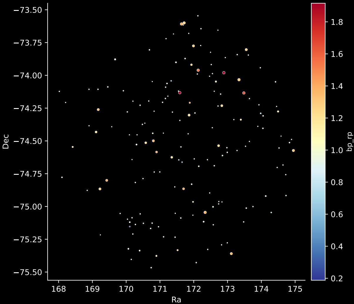
GALAH DR4 Field: [7205] Stars: 167
