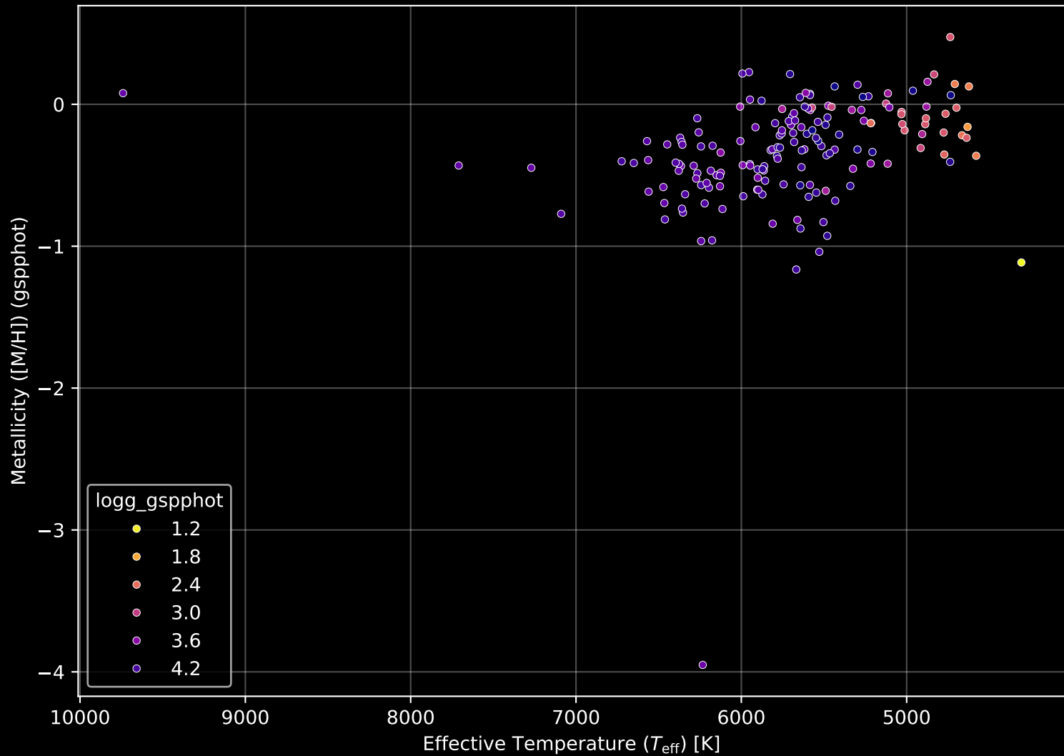
GALAH DR4 Field: [7205] Stellar Population Parameters (n= 167)
